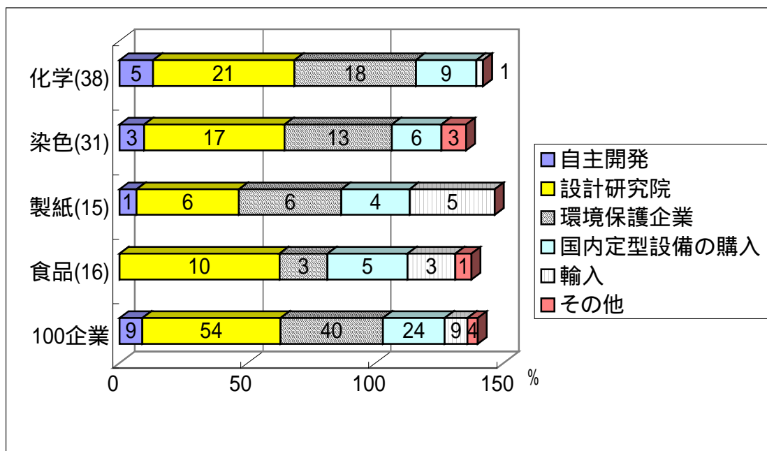
図8 排水処理施設の技術供給源
