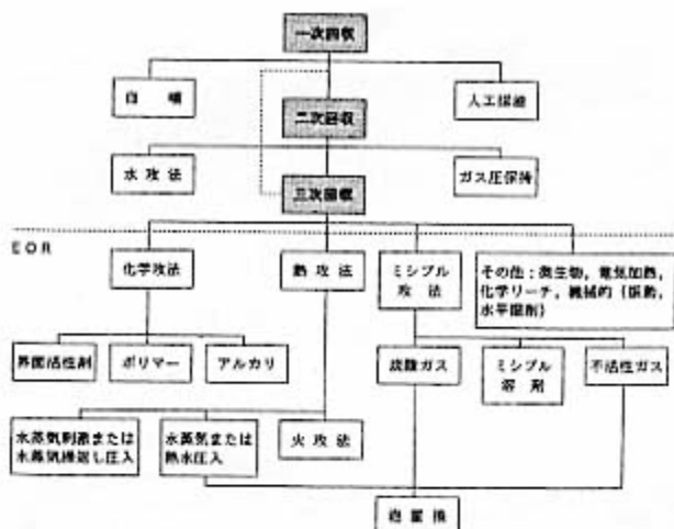
図1 石油の回収法
